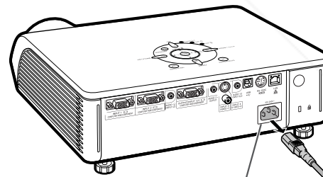
AC socket
