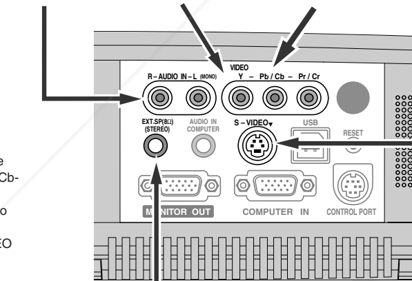
Terminales del proyector
