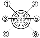
DIN 8 clavijas Aspecto exterior
