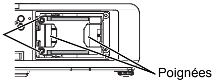
Vis de fixation de l'Unité de la lampe
