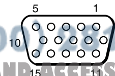
D-sub 15pin (Male)
